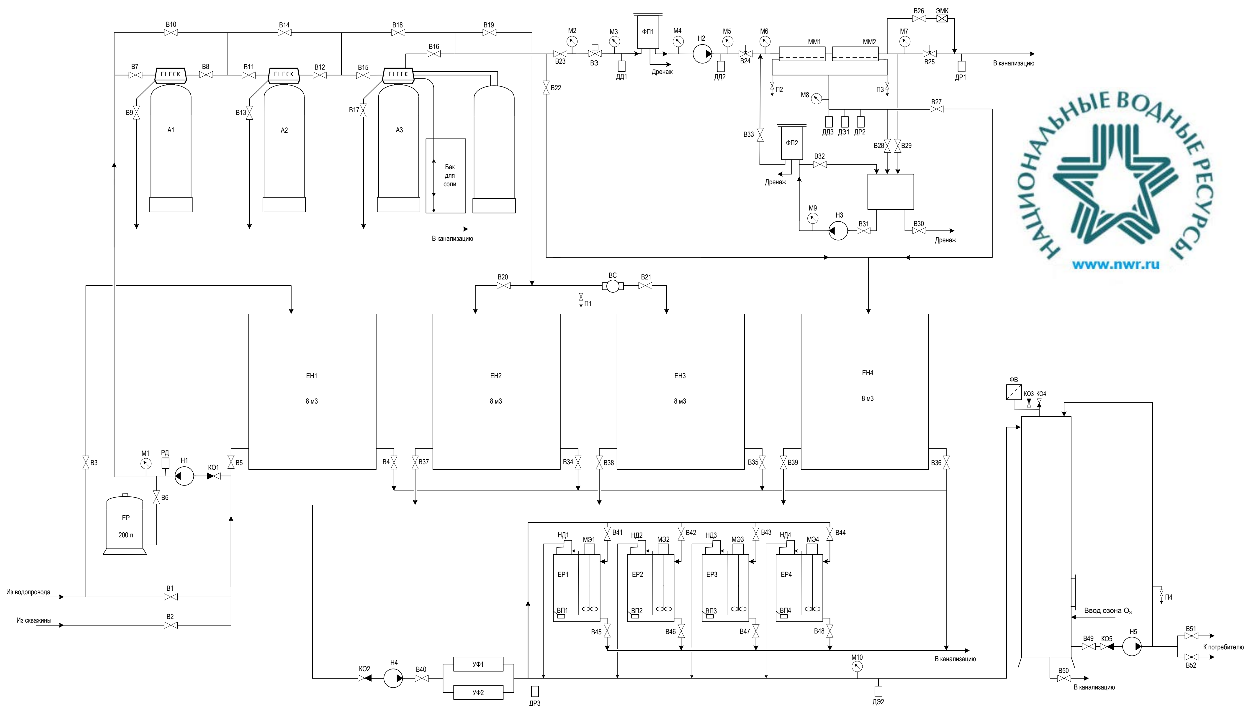
Схема водоподготовки для линии розлива безалкогольных напитков Братского пивоваренного завода.
